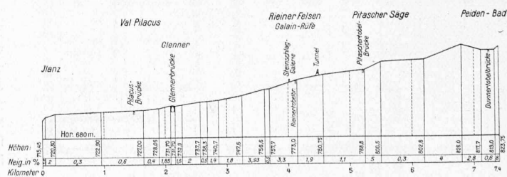
Abb. 2. Längenprofil der Glennerstrasse. — 1:80 000 f. H., 1:800 f. L.
