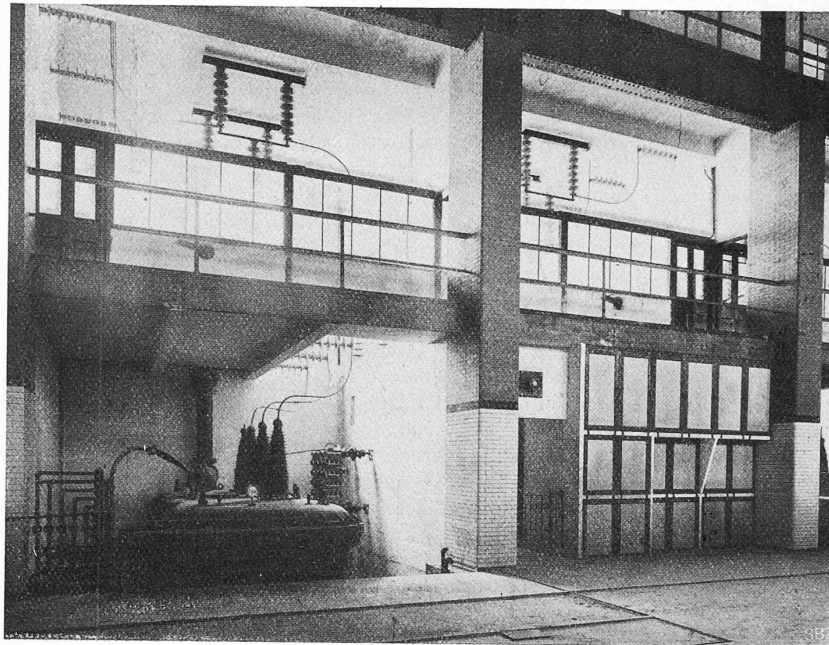
Abb. 33. Transformatoren-Raum der Zentrale.
