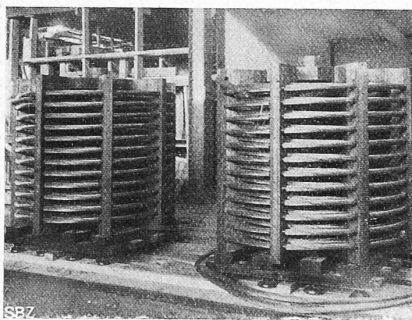
Abb. 32. Reaktanz-Spulen.
