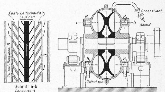
Abb. 8. Schematische Schnitte.
