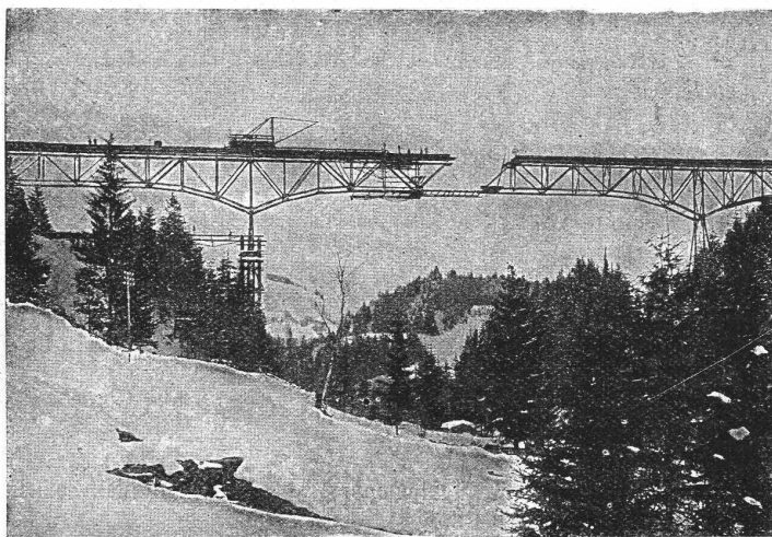
Hochbrücke über den Argentobel (Allgäu); Freimontage der Mittelöffnung.
