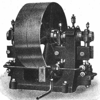
Dreifache Presspumpe
