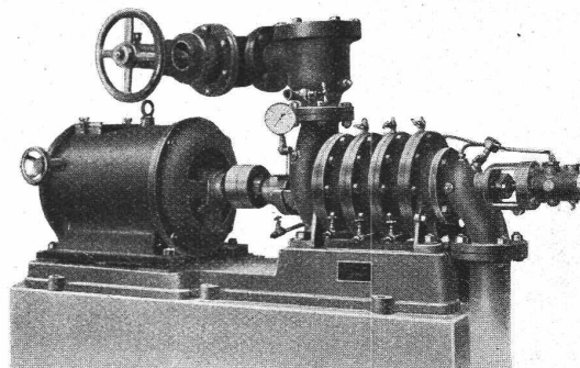
Viersstufige Hochdruckzentrifugalpumpe
