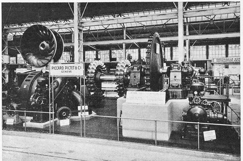
Abb. 2. Société Anonyme des Ateliers Piccard, Pictet & Cie., Genève. (Das Francis-Laurens links oben gehört zum Stand von Th. Bell & Cie.)
