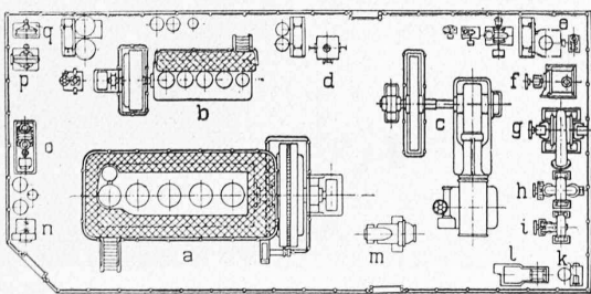
Abb. 2. Ausstellung von Gebr. Sulzer, A.-G. — Grundriss 1 : 300.
