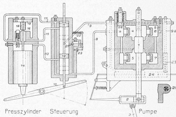
Abb. 3. Schematische Darstellung der Nietmaschine System Spillmann.
