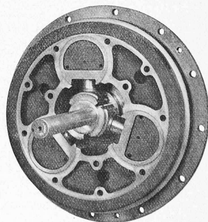
Abb. 18. Kolben-Oelpumpe.
