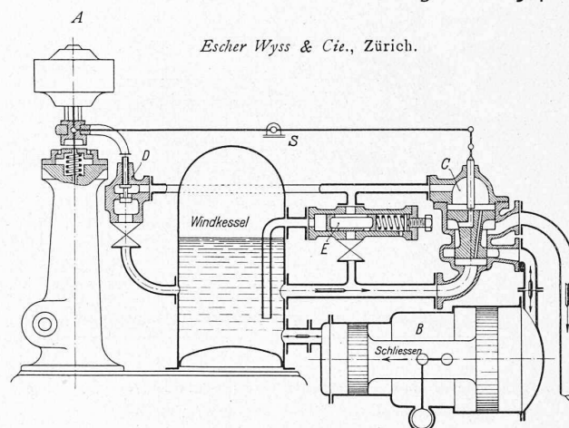
Abb. 20. Schema zu nebenstehender Abb. 21.
