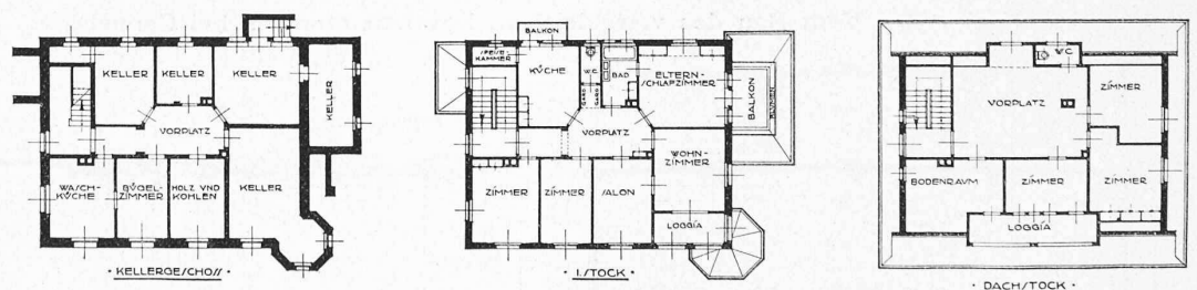
Abb. 1 bis 4. Grundrisse.
