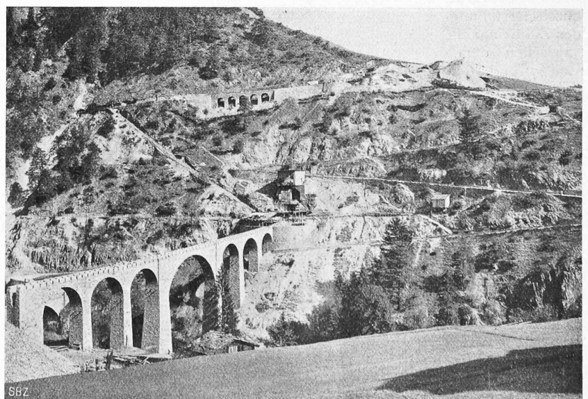
Abb. 12. Grenchols-Viadukt bergwärts gesehen, mit Einfahrt in den Kehrtunnel. Oberhalb Austritt der Bahn aus diesem.
