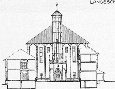
QUERSCHNITT DURCH DEN HOF.
