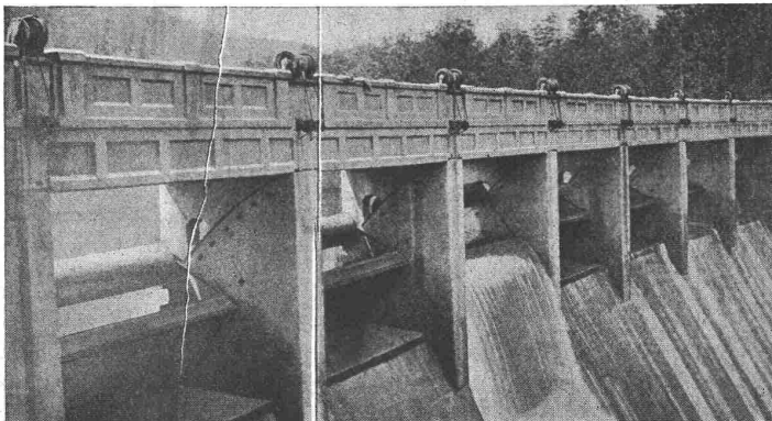
Automatische Ueberfallwehre auf einer Talsperre in Tallulah Falls (U. S. A.)
