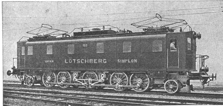
2500 PS-Einphasen-Lokomotive der Lötschbergbahn.
