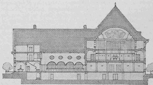
Querschnitt. — Masstab 1:600.
