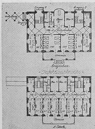
Grundrisse vom Erdgeschoss und I. Stock des Absonderungs- und Rekonvaleszentenhauses. — 1:800.
