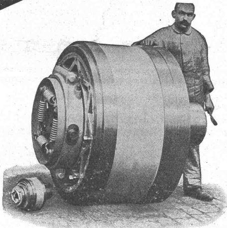
Bann Kupplung Nr. 12 für 600 PS geliefert in eine Zementfabrik.
