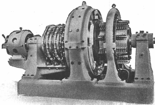
Einanker-Umformer.
