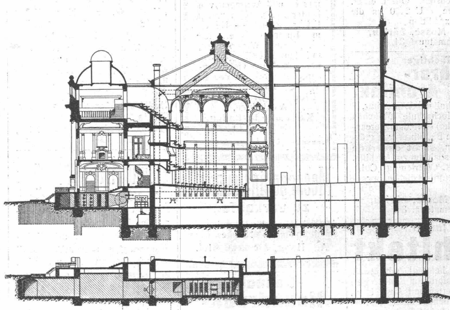
Abb. 2 Platzbedarf einer Anlage nach altem System
