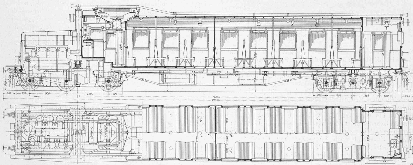
Abb. 1 (oben) Ansicht des Diesel-elektrischen Triebwagens. — Abb. 3 (darunter) Längsschnitt und Grundriss, etwa 1:110.
