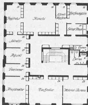
Abb. 12. 1. Stock. — 1 : 500.
