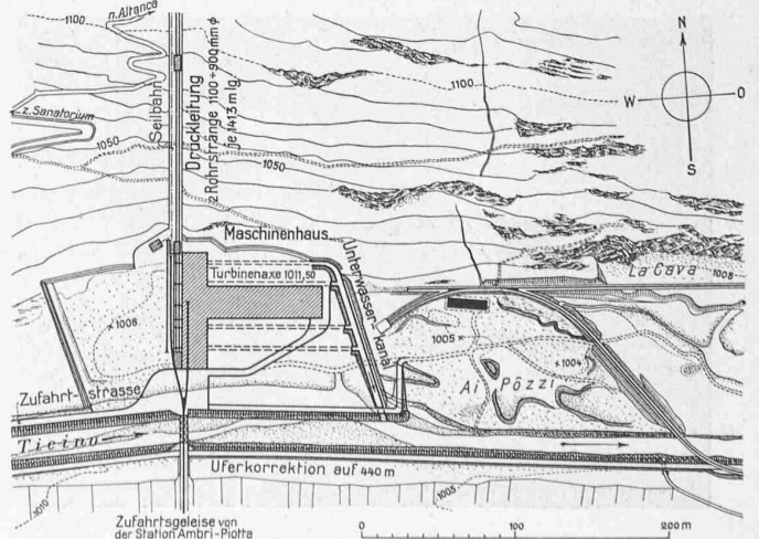
Abb. 16. Lageplan des Maschinenhauses. — 1 : 5000.
