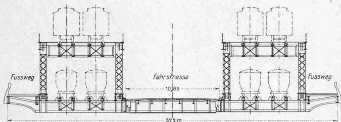
Abb. 13. Fahrbahntafel der Manhattan-Brücke.
