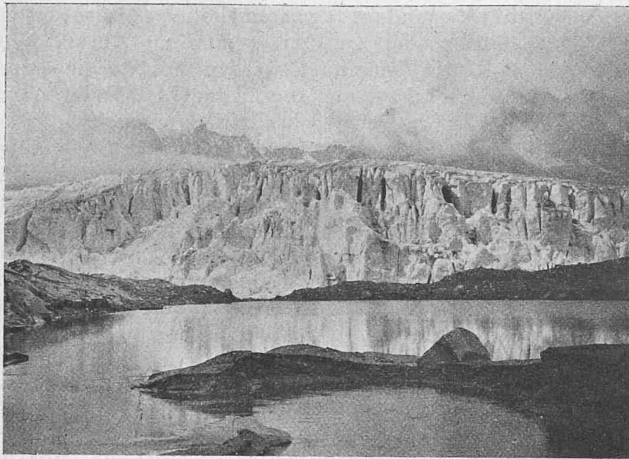
Abb. 9. Blick vom Ostende des kleinen, durch die alte Endmoräne der Gletscherzunge gebildeten Seelins im Becken des ausgelaufenen Hintersees (12. September 1913).
