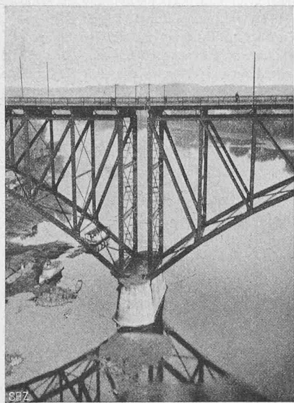
Abb. 64. Mitteljoche auf dem Strompfeiler der Fort Snelling-Brücke.
