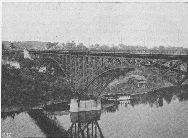
Abb. 63. Fort Snelling-Brücke, Spannweite 2 x 111 m, über den Mississippi bei San Paul (Minn.).
