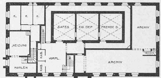
Westfassade 1:400. — Entwurf Nr. 21 „Nervus rerum“ I. Orientierung wie bei Entwurf Nr. 72. — Grundrisse 1:400.
