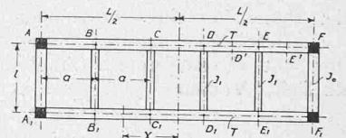
Grundriss.
