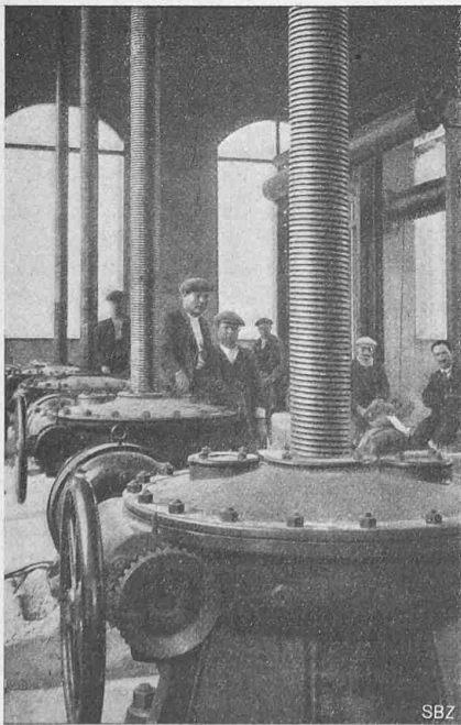
Abb. 27. Schütten-Hubspindeln mit Motor- und Hand-Antrieb.
