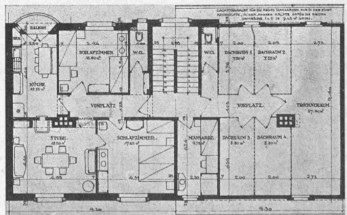
2. Rang, Entwurf Nr. 5 „Platzbildung“. — Architekten Kündig &amp; Oetiker, Zürich. — Typ Zurlindenstrasse, Grundrisse. — Masstab 1:200.
