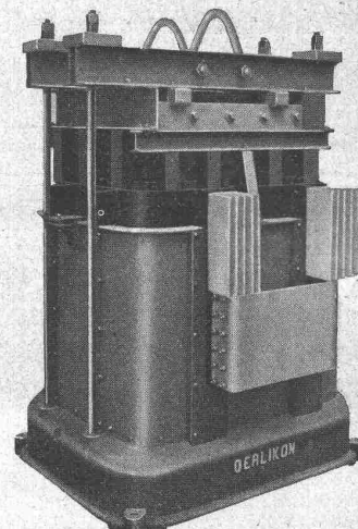
Einphasenwechselstrom-Transformator mit künstlicher Luftkühlung. Leistung 1500 kVA, 4000 Volt primär, 100 Volt und 15000 Ampère sekundär, 50 Perioden.
