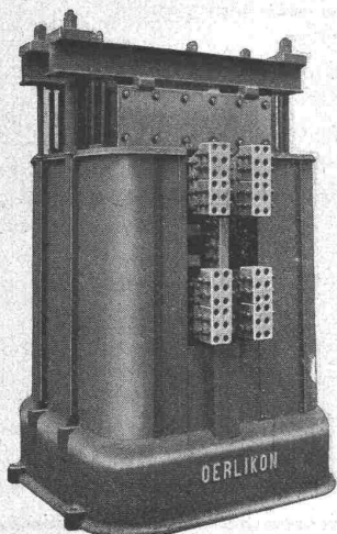
Einphasenwechselstrom-Transformator mit künstlicher Luftkühlung. Leistung 6000 kVA, 10000 Volt primär, 150 Volt und 40000 Ampère sekundär, 50 Perioden.
