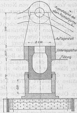
Abb. 7. 3000 t-Press. — Schnitt 1:75.
