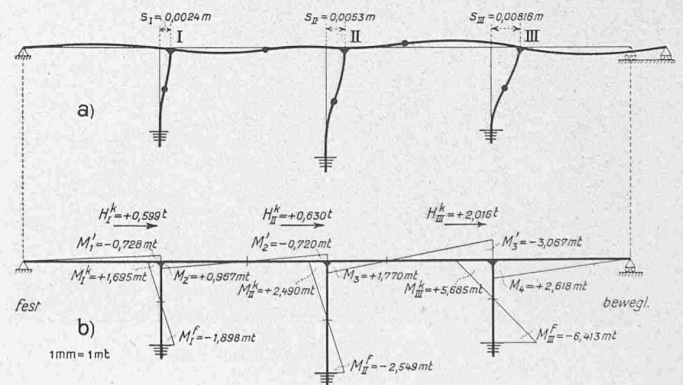
Abb. 9. Momente und Horizontalschübe am Rahmen mit festgehaltenem Balken infolge Temperatur-Erhöhung von \pm 20^\circ \text{ C} .
