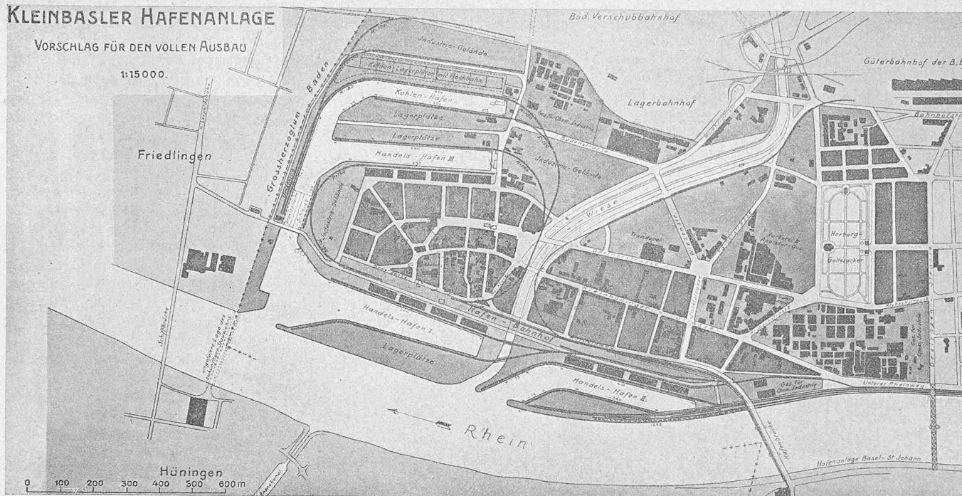
Abb. 5. Genereller Entwurf des Basler Ingenieur- und Architekten-Vereins zum Vollausbau des Rheinhafens in Kleinhünningen. — 1 : 15 000.
