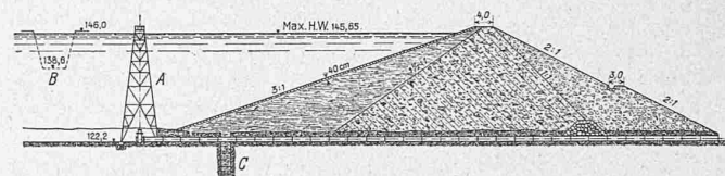
Abb. 66. Querschnitt des Dammes Nr. 3. — Masstab 1:1500.
