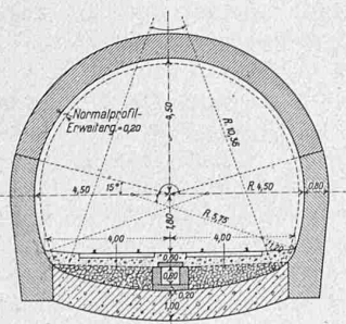
Abb. 27. Verstärktes Tunnelprofil, 1 : 250.
