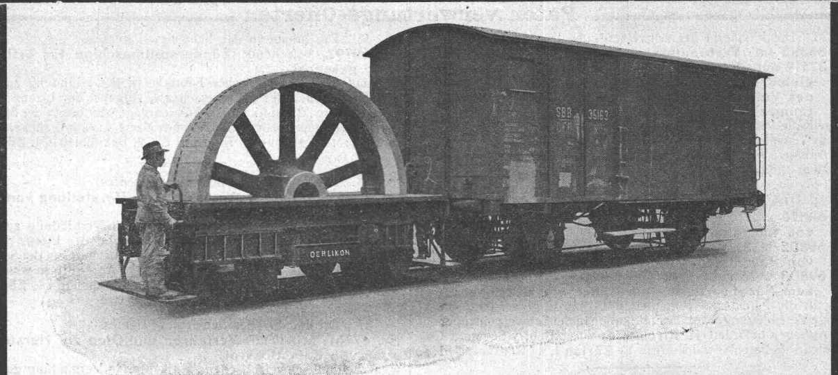
Akkumulatoren-Plattformwagen für Transporte in Werkstätten und für Verschiebedienst
