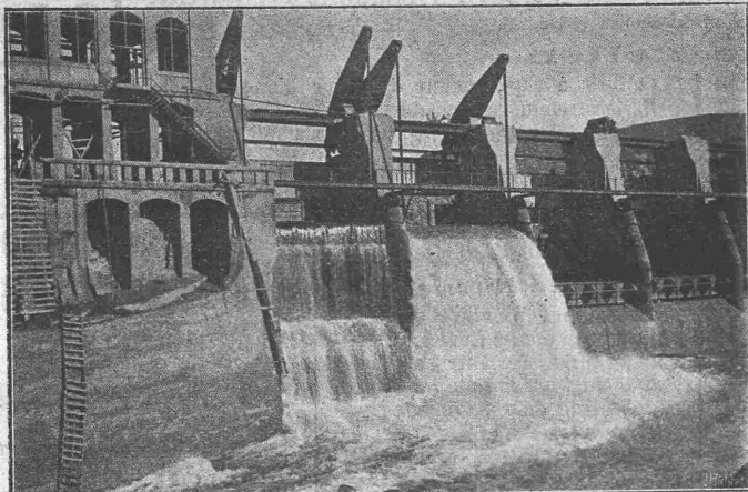
Zwei von sieben selbststättigen Ueberfallwehren, je 10,0 m breit, 6,00 m hoch, der Stauanlage Riegos y Fuerza del Ebro S. A. Tremp (Spanien).
