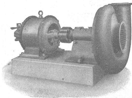
Einstufiger Hochdruck-Zentrifugalventilator
