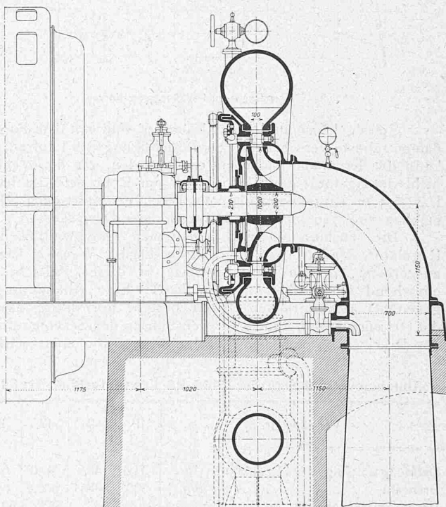
Abb. 1. Spiral-Francisturbine mit fliegend aufgesetztem Laufrad für 2500 PS bei 500 Uml/min, gebaut von Escher Wyss & Cie. — 1 : 40.
