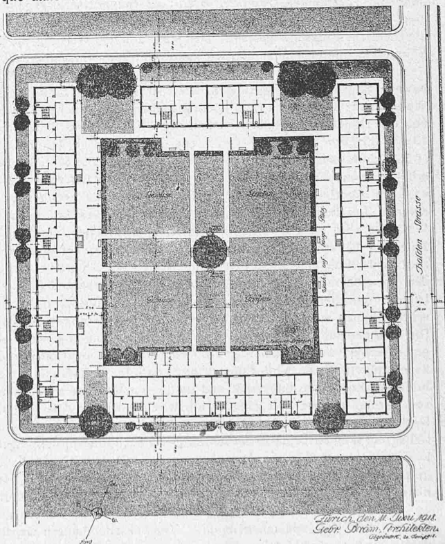
Abb. 1. Wohnhäuser-Gruppe auf dem „Rebhügel“ in Zürich-Wiedikon. — Arch. Gebr. Bräm, Zürich. — Lageplan 1 : 1000.
