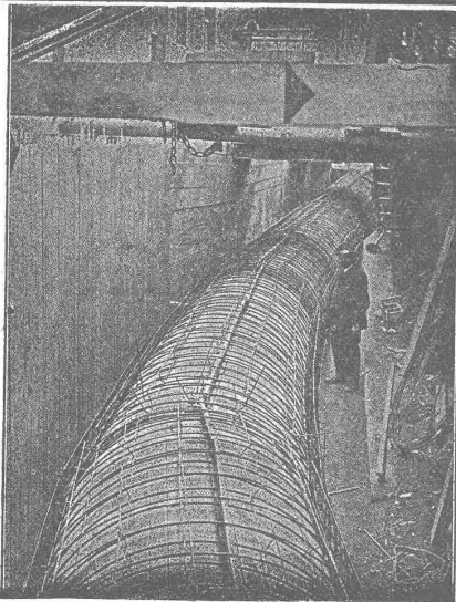
Druckrohr in Eisenbeton von 2 m Durchmesser der Wasserkraftanlage Stöcklin & Cie., Basel, 1916/17.
