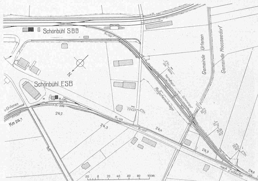
Abb. 28. Station Schönbühl-E. S. B. mit Rollschemel-Anschluss an Schönbühl-S. B. B. — 1:4000.
