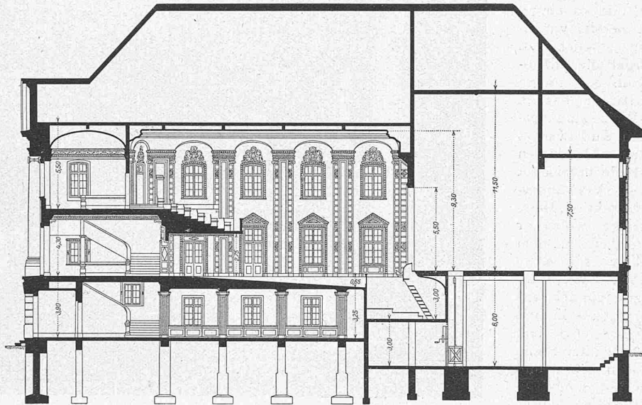
Abb. 4. Längsschnitt. — Masstab 1:300.
