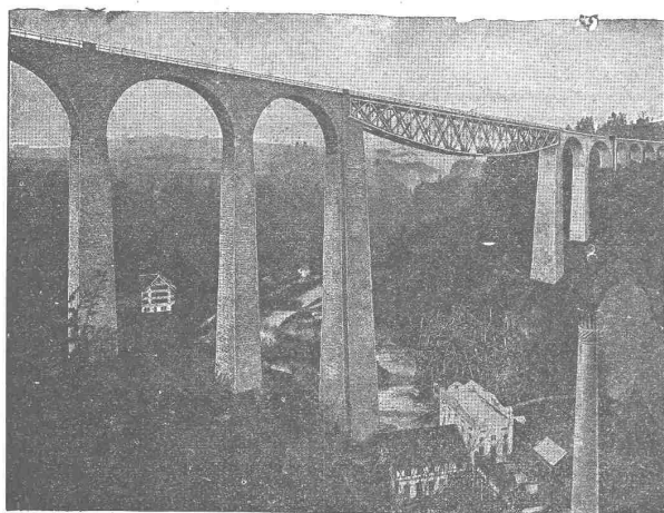
Sitterviadukt mit zur Hälfte abgebrochenem Gerüsturm.
