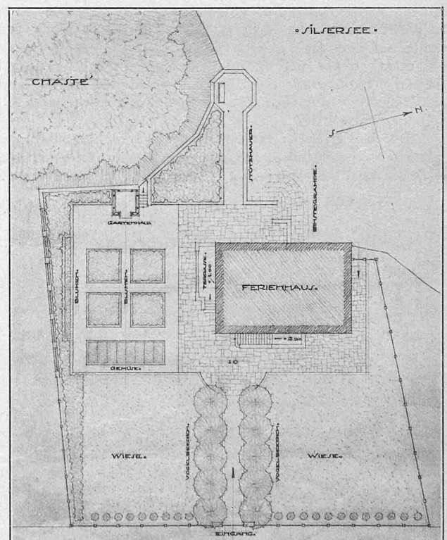
Abb. 1. Ferienhaus Bartuns am Silsersee. — Lageplan 1:500.
