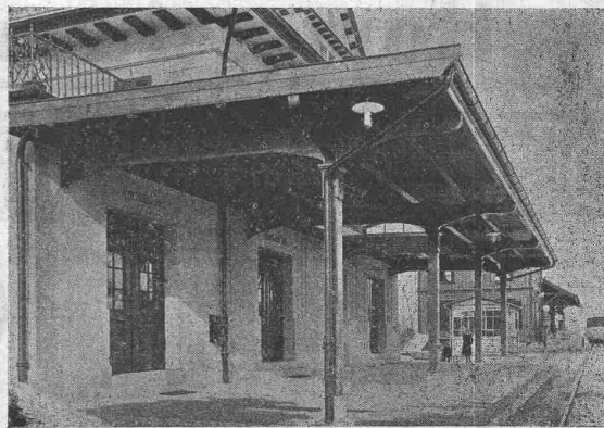
Perrondach Oberwinterthur.
