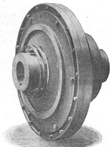
Elektromagnetische Reibungskupplung. Patent.
