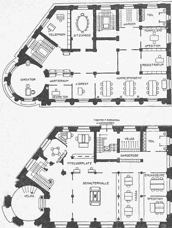
III. Rang (2000 Fr.) Entwurf Nr. 7 „Wilson“. — Architekten A. Jeanmaire & Boillat in Biel. — Grundrisse 1:400 und Ansicht vom Zentralplatz aus
