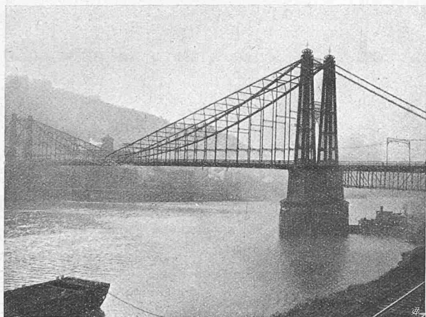
Abb. 4. Steife Hängebrücke über den Monongahela in Pittsburg.
