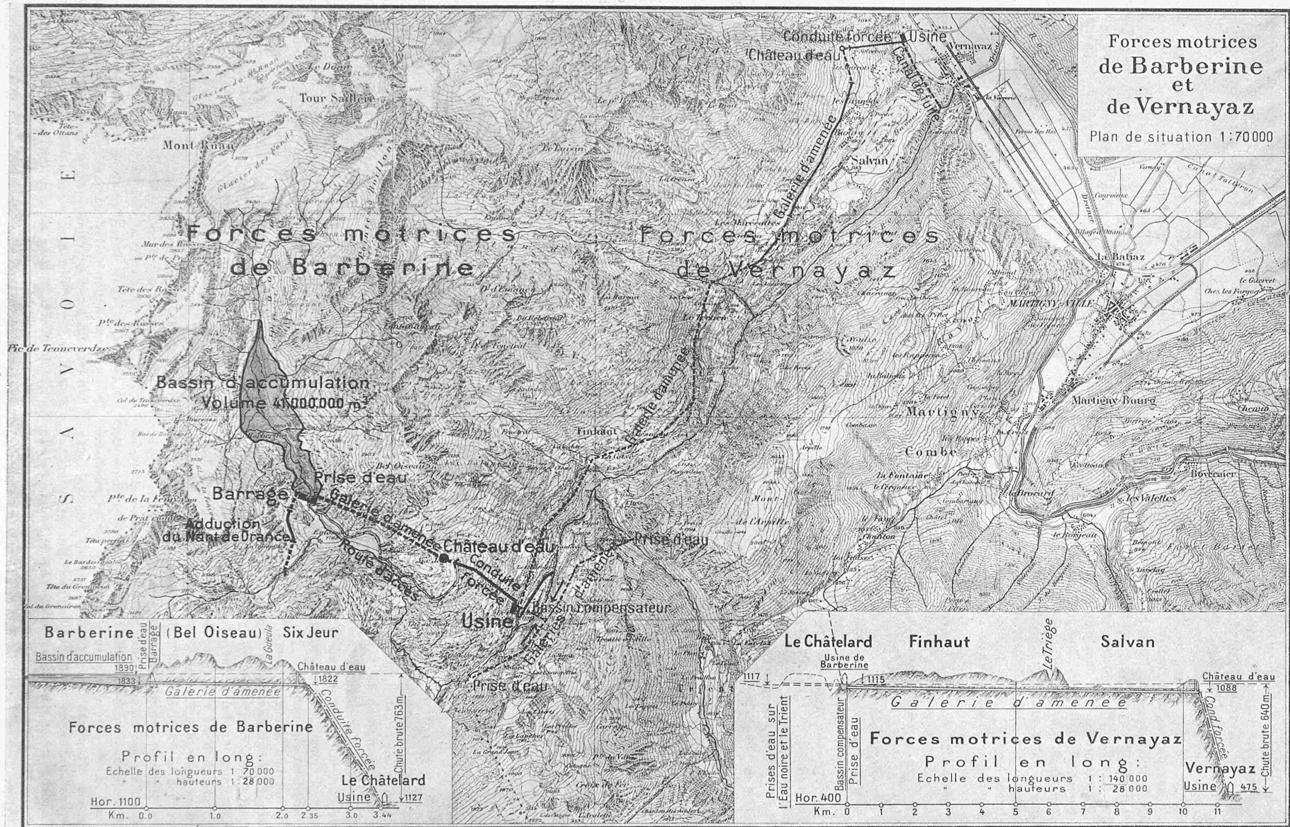
Übersichtskarte 1:70 000 und generelle Längenprofile 1:70 000 / 1:28 000 (Barberine) bzw. 1:140 000 / 1:28 000 (Vernayaz). — Mit Bewilligung der Schweiz. Landestopographie.
