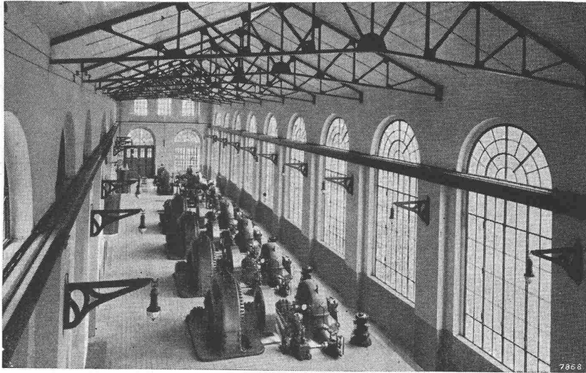
Wasserkraftwerk Cairasca und Diveria. 4 Einheiten von je 3000 kW, und 2 Einheiten von je 1200 kW.
