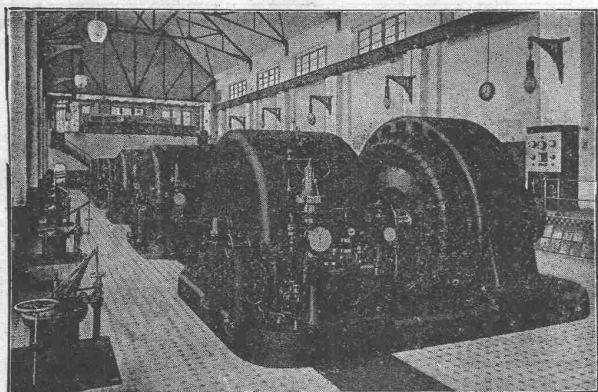
Löntschwerk 70000 PS
